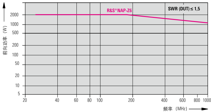
R&S ® NAP-Z6探头的最大持续功率等级（调制信号峰值包络功率（PEP））
