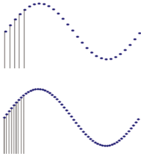
图 26. (上) 水平分辨率低; (下) 水平分辨率高。水平或定时分辨率是指边沿、周期时间或脉宽可以变动的最小时间增量。
