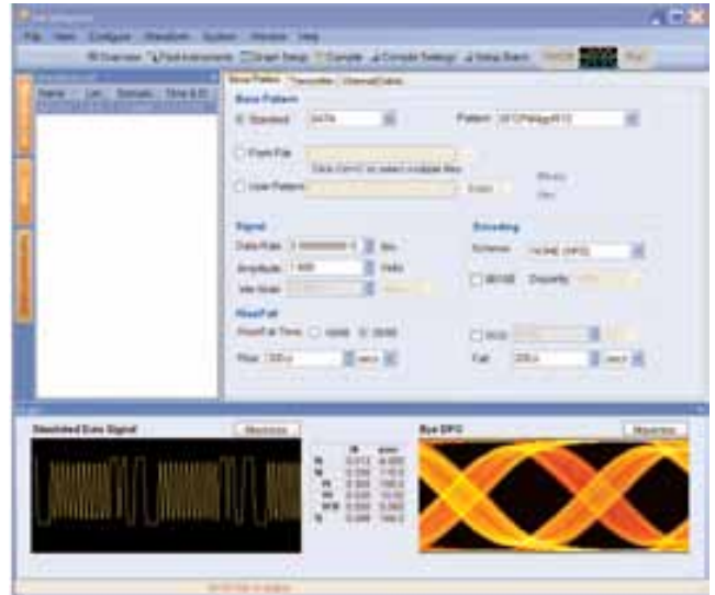
图 37. 预加重的标准 SATA 波形。
