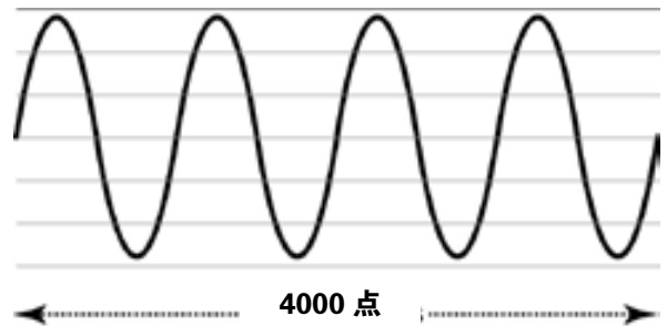
图 23. 通过使用四个存储的波形和一个 100 MHz 时钟，生成了一个 100 kHz 信号。
