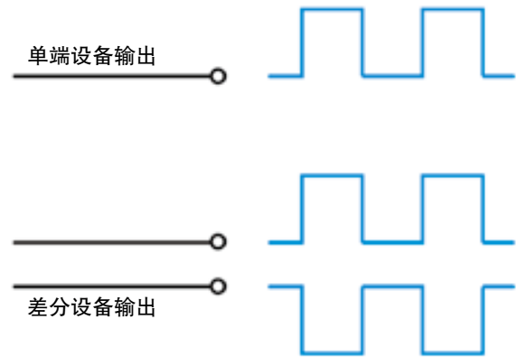
图 7. 单端和差分信号
