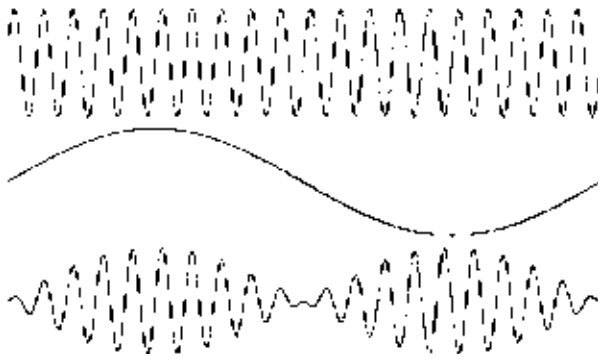
图 12. 幅度调制
