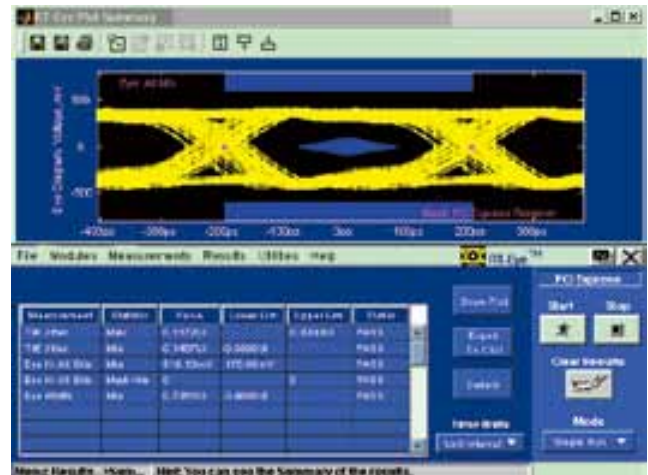
图 42. DTG 使用小的定时位移模拟抖动。
