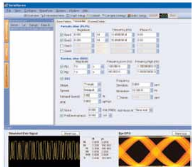
图 38. SerialXpress 可以轻松生成损伤信号。
