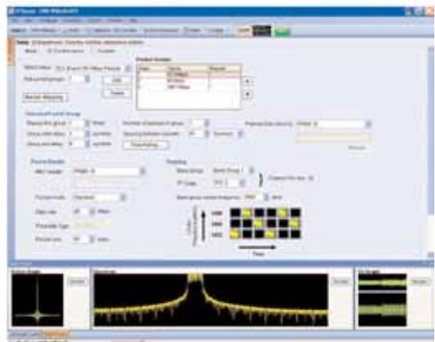
图 40. 使用 RFXpress 创建的复杂的 UWB 波形。
