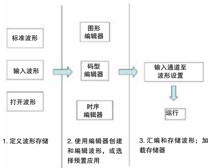
图 35. 使用 AWG 创建波形的基本步骤。
