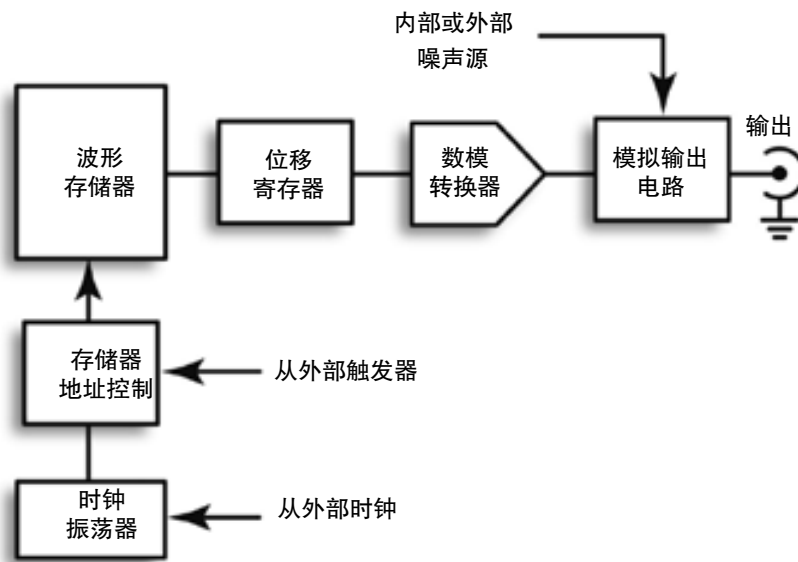
图 18. 任意波形发生器的结构 (简图)。
