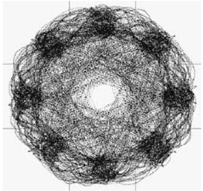
图 15. 正交调制。
