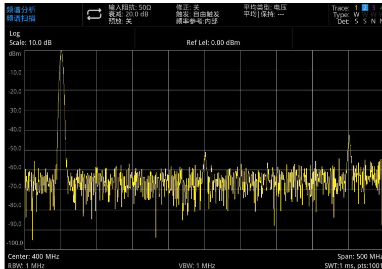
图 3-16 谐波失真
