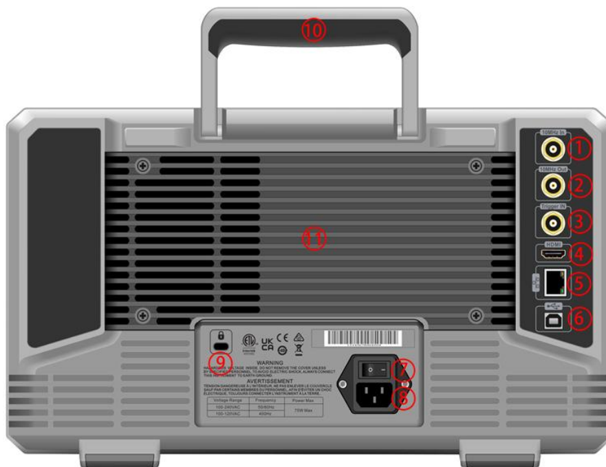
图 1-3: 后面板
