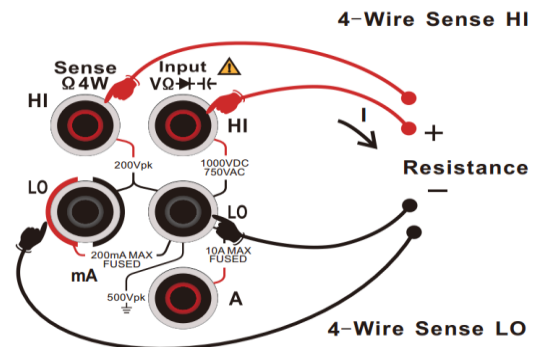
图 2-16 四线电阻测量连接示意图
