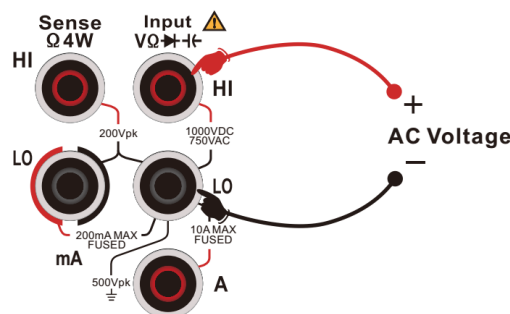
图 2-9 交流电压测量连接示意图
