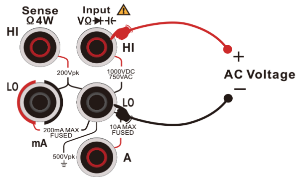
图 2-20 信号频率测量连接示意图
