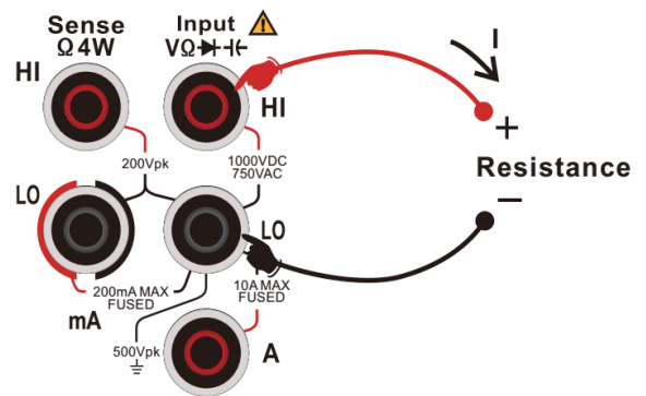
图 2-14 二线电阻测量连接示意图
