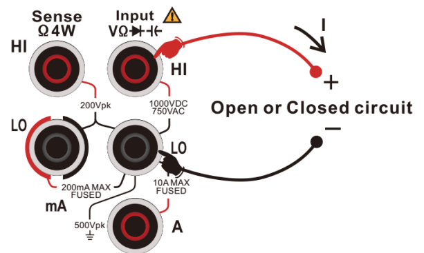
图 2-24 连通测量连接示意图
