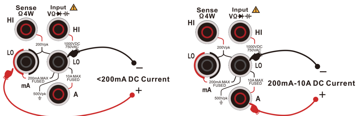
图 2-7 直流电流测量连接示意图
