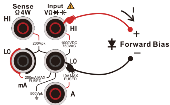
图 2-26 二极管测量连接示意图
