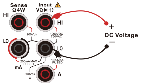
图 2-5 直流电压测量连接示意图
