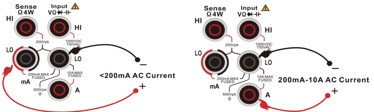
图 2-12 交流电流测量连接示意图
