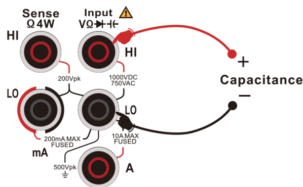
图 2-18 电容测量连接示意图
