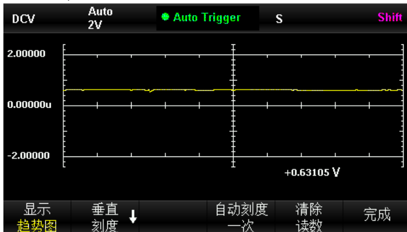
图 2-49 趋势图显示模式
