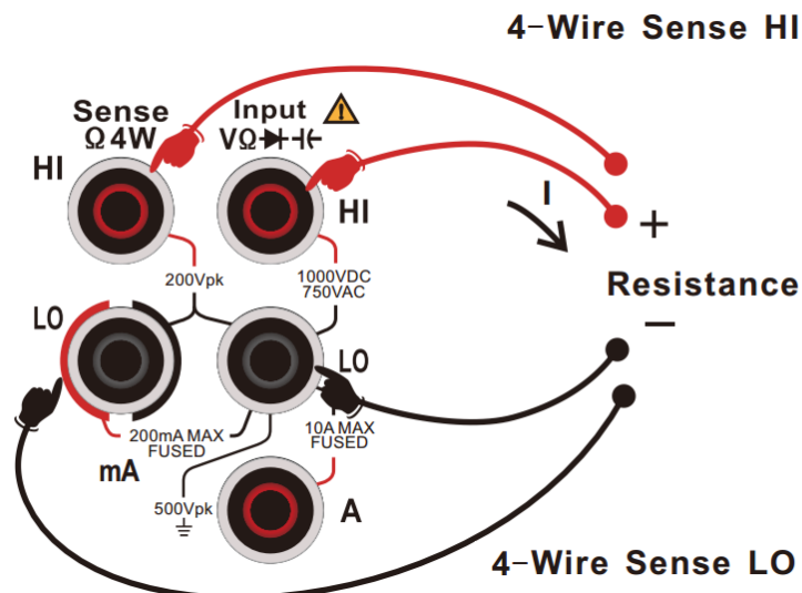
图 2 - 23 四线电阻测量连接示意图
