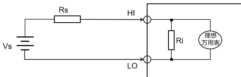
图 3 - 1 误差来源示意图
