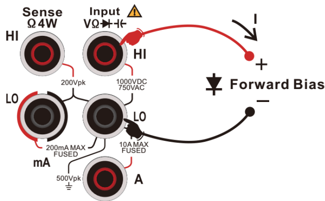
图 2 - 33 二极管测量连接示意图
