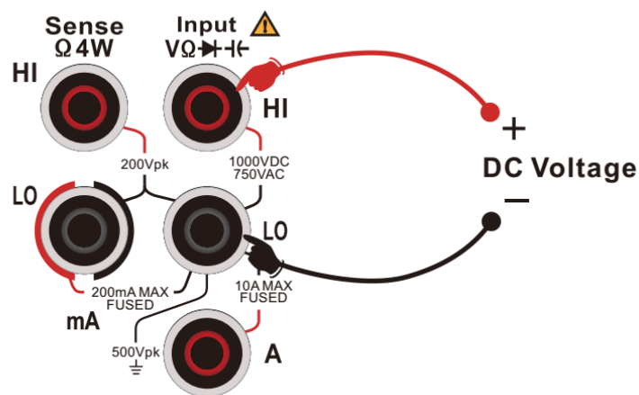
图 2 - 11 直流电压测量连接示意图
