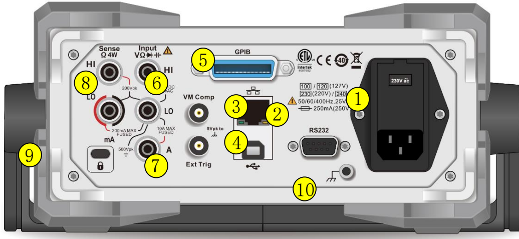
图 1 - 6 后面板示意图
