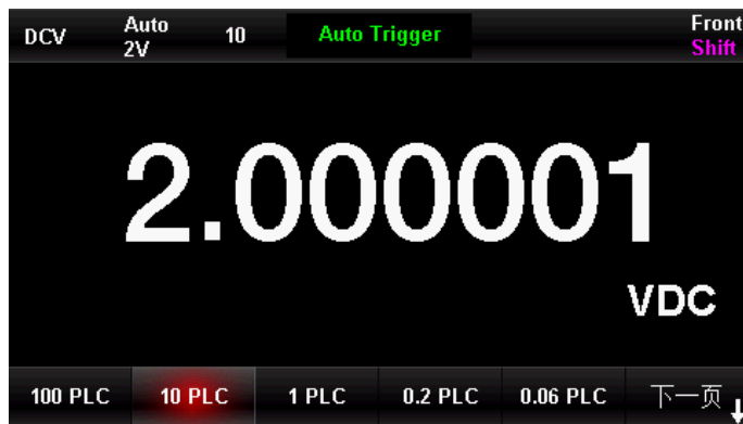
图2-3积分时间选择菜单
