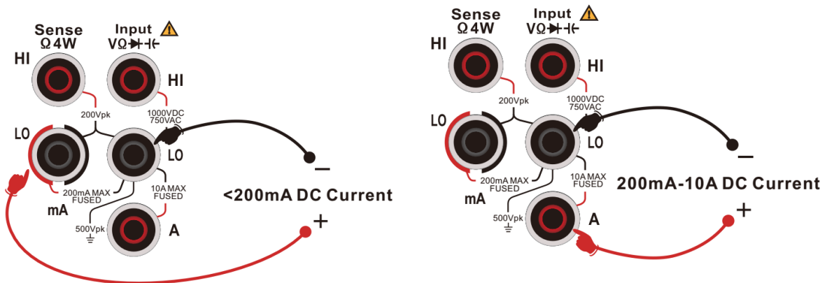
图 2-13 直流电流测量连接示意图
