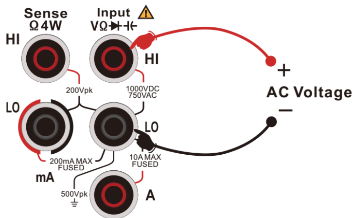
图 2-15 交流电压测量连接示意图
