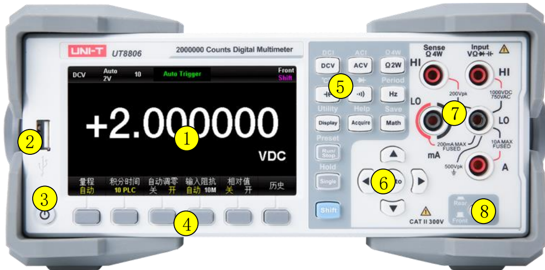
图 1 - 5 前面板示意图
