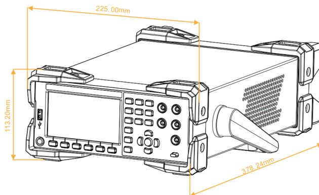
图 1-4 外观尺寸
