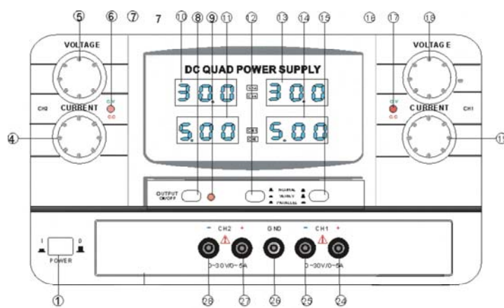
图 3-1 前面板示意图及说明
