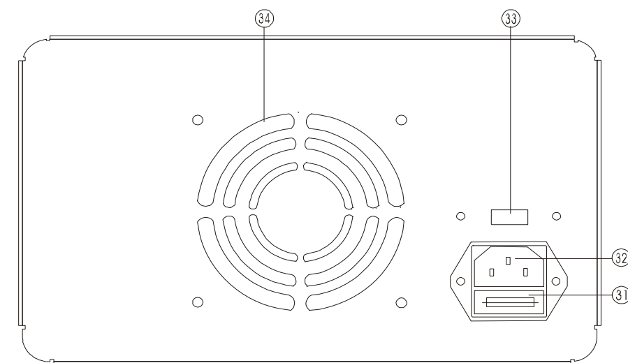
图 3-2 后板图及说明
