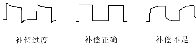
图1-6 探头补偿调整
