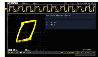
磁性分析
