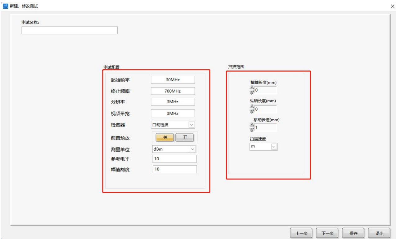
图 7 设置频谱采集参数、扫描范围和扫描速度
