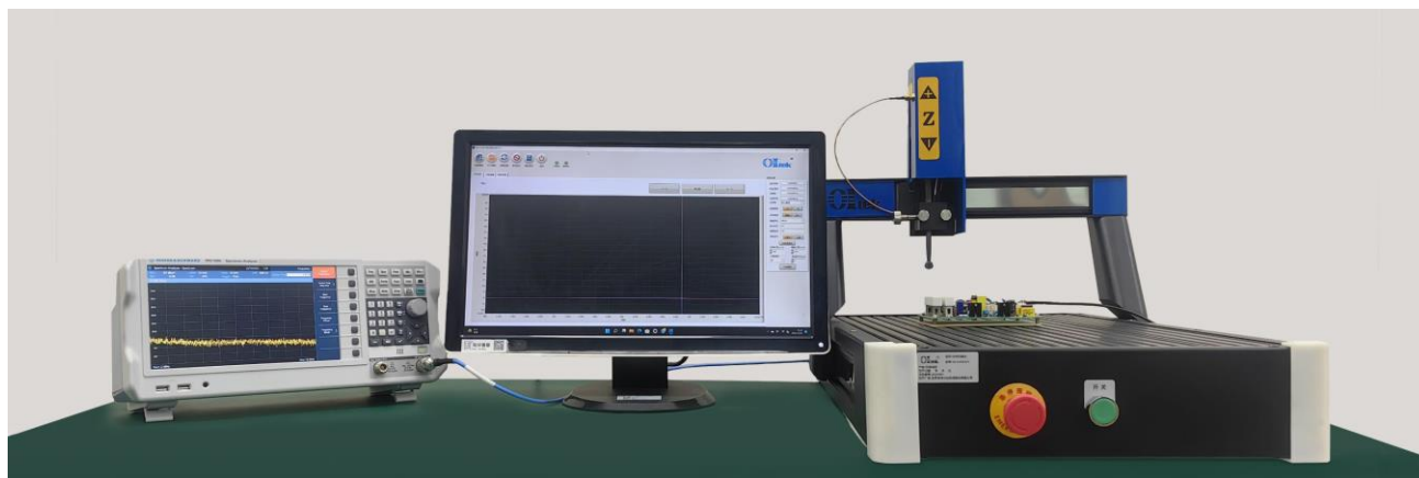
图 20 OI-EAS 系列电磁干扰扫描仪（标配不包含频谱分析仪、EMI 接收机、近场探头、前置放大器和电脑）
