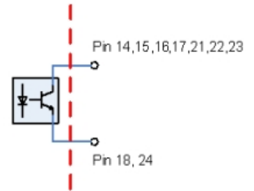
Photo coupler output CKT
