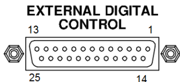
圖 2-8 外部數位控制連接埠
