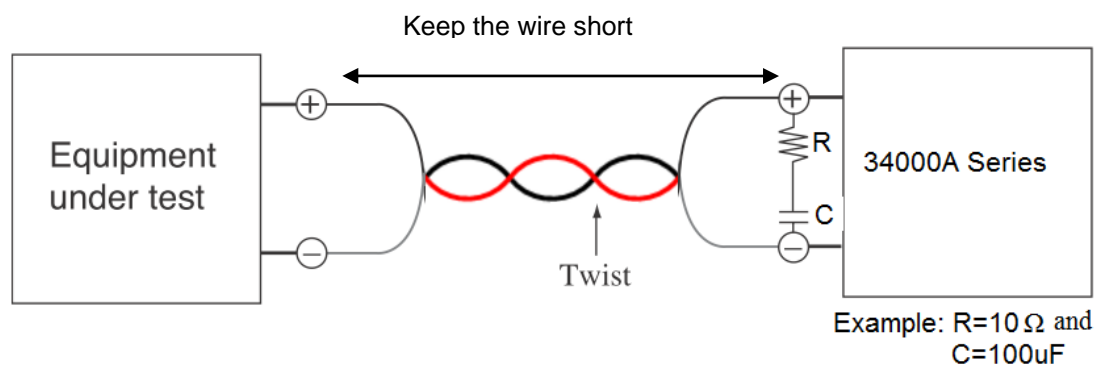
圖 2-12 接線長度
