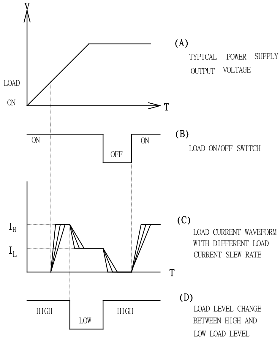
圖 2-10 負載電流波形與 LOAD ON/OFF 開關
