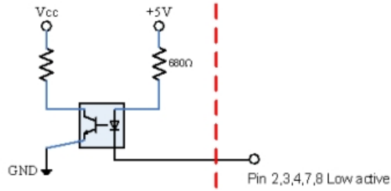
Photo coupler input CKT
