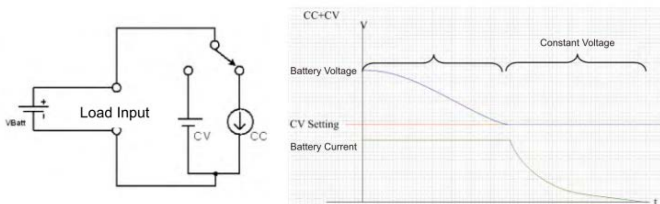
圖 5-8 CC+CV操作模式之應用
