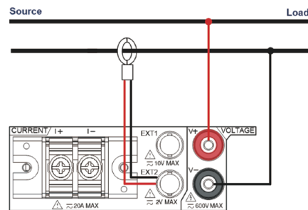
外部电流感应端子
