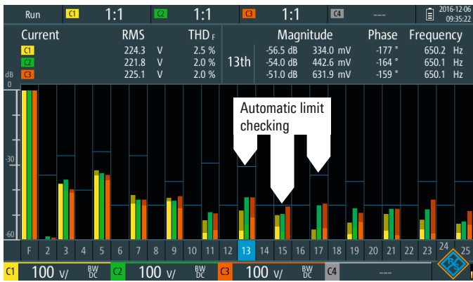
具有自动限值检查功能的三相系统的谐波分析
