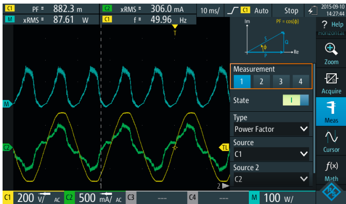
使用自动测量功能测量电子负载的功率因数
