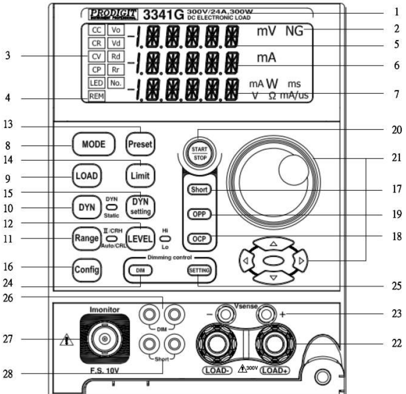
圖 3-1 前面板圖
