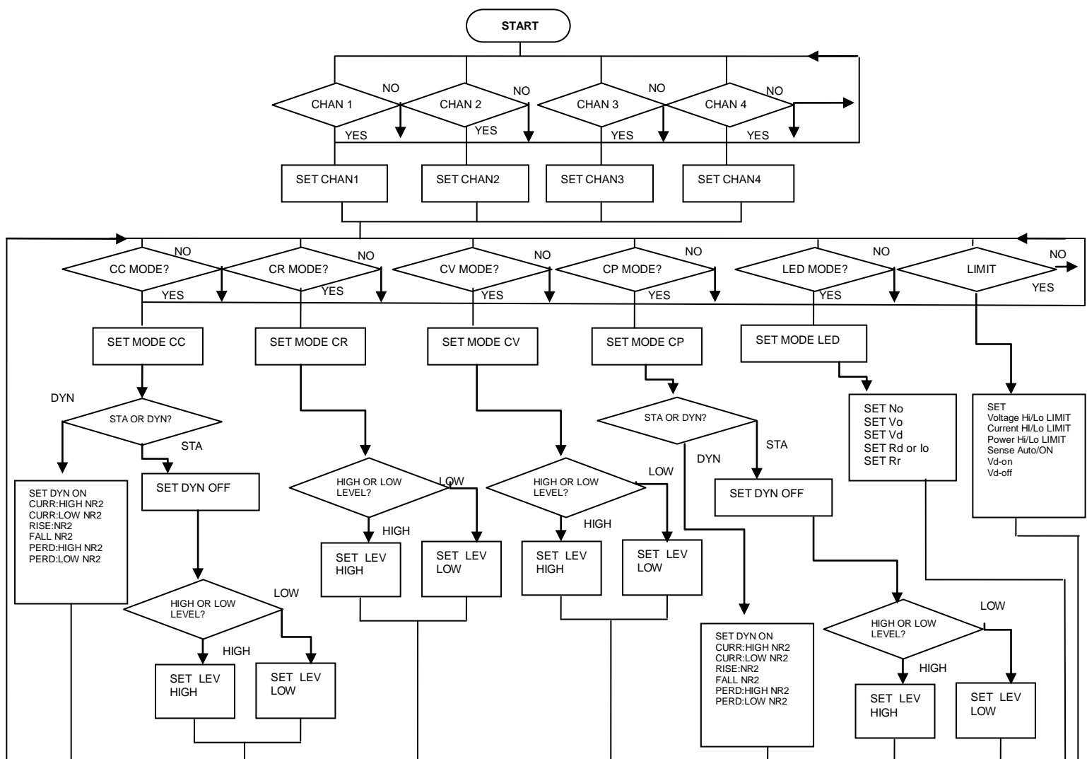
圖 2-3 3341G 系列電子負載操作流程圖
