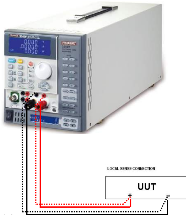
圖 4-2 遠地電壓檢知連接圖
