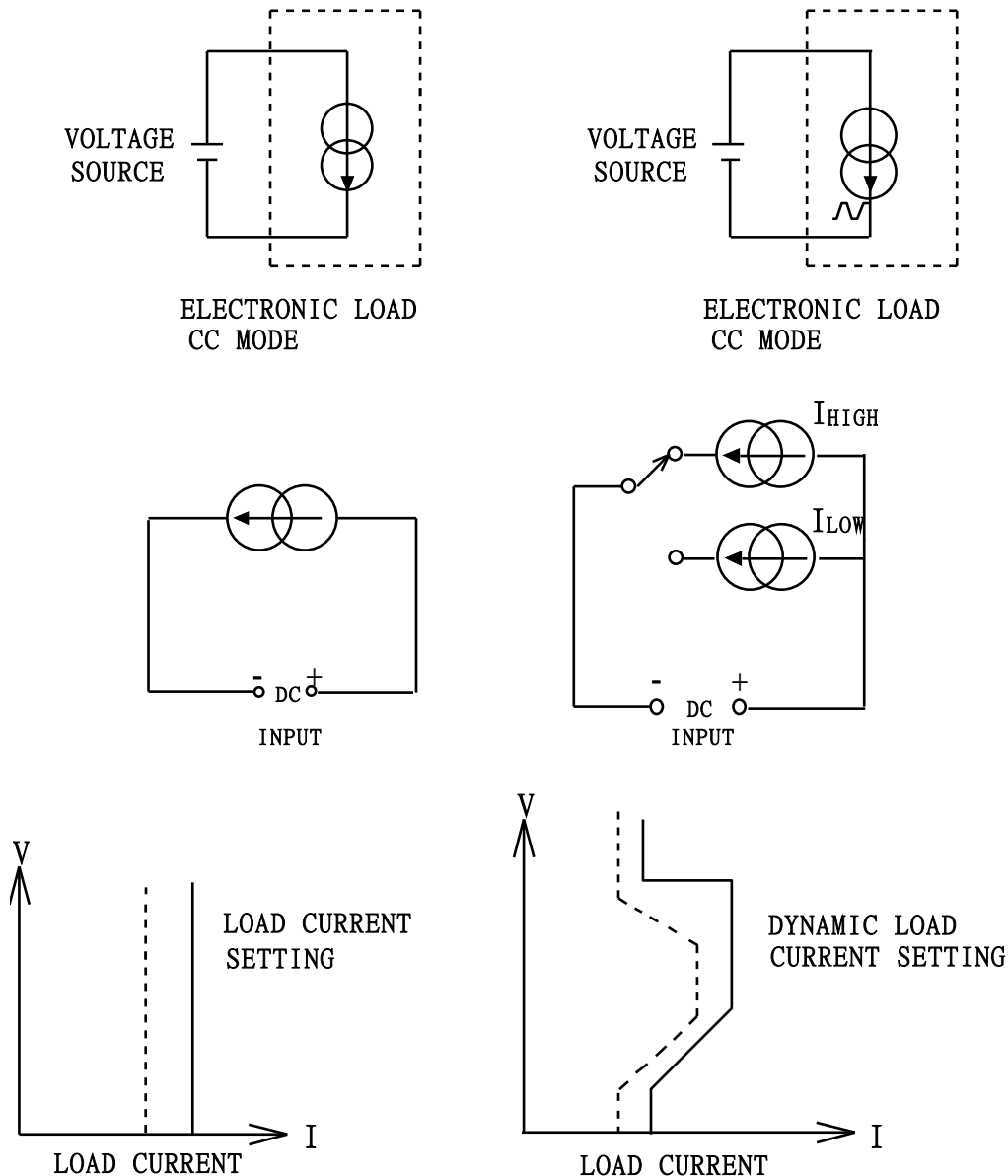
圖 4-3 固定電流操作模式之應用
