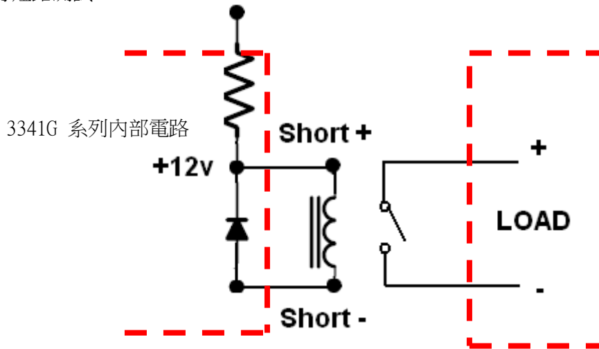
圖 4-17 short 測試連接圖
