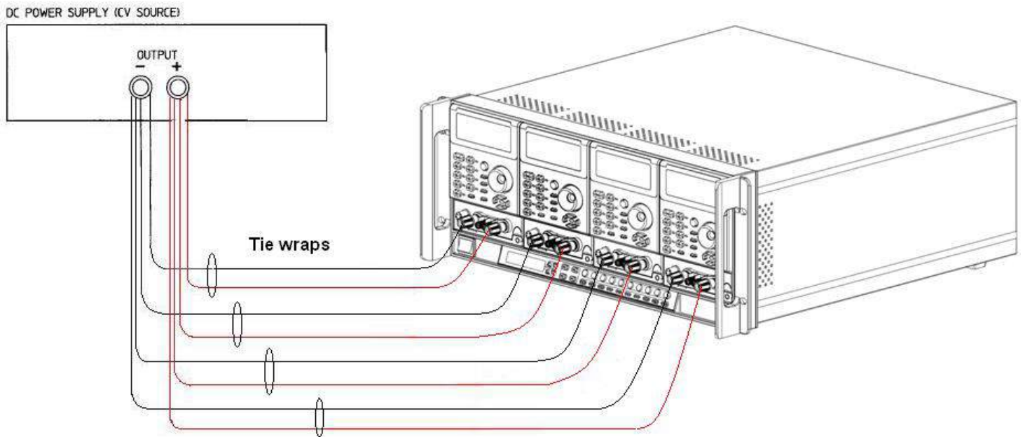
圖 4-14 電子負載多組並聯之連接圖
